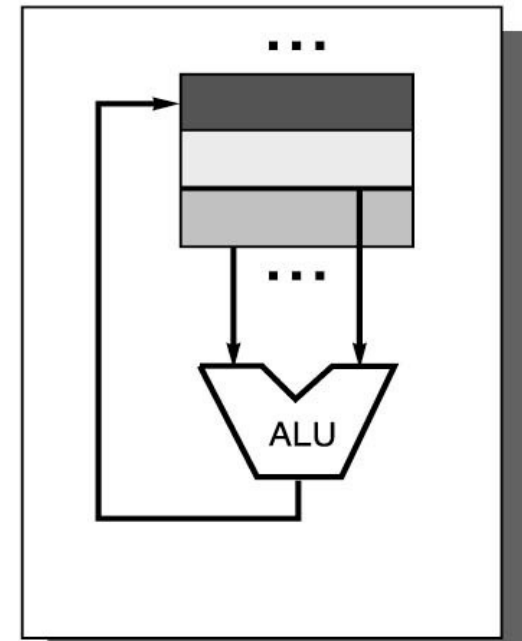
(d) Register-register/load-store
